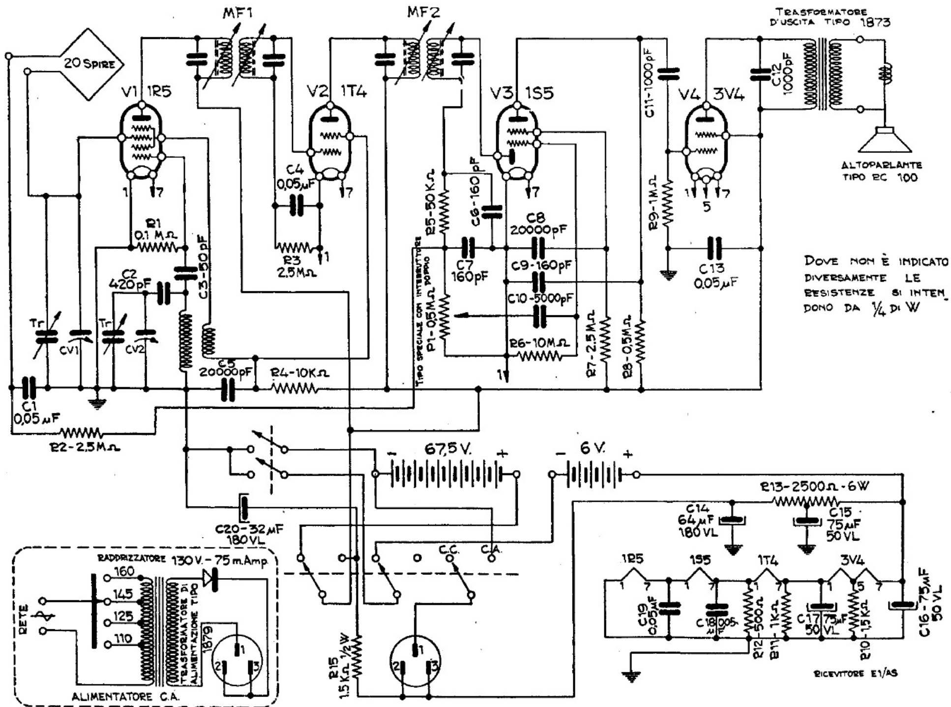
NOVA RADIO - Modd. AS e E1 - Portatile alimentato con pile e adatto per funzionare anche con la tensione alternata della rete luce. Media frequenza 465 ke.
